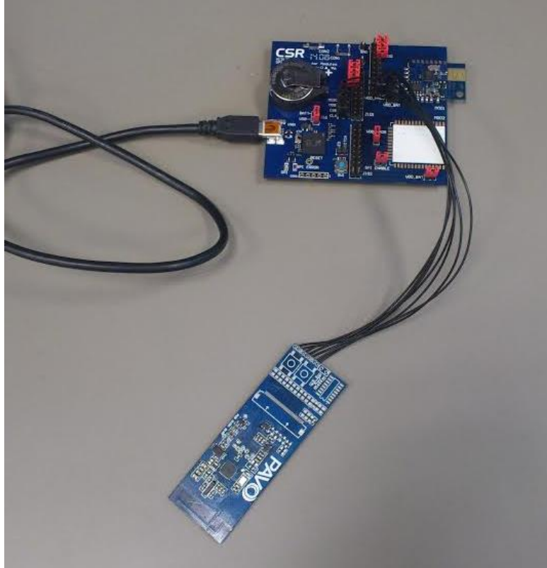
Şekil 4 - Tasarlanan PCB ve geliştirme kiti
