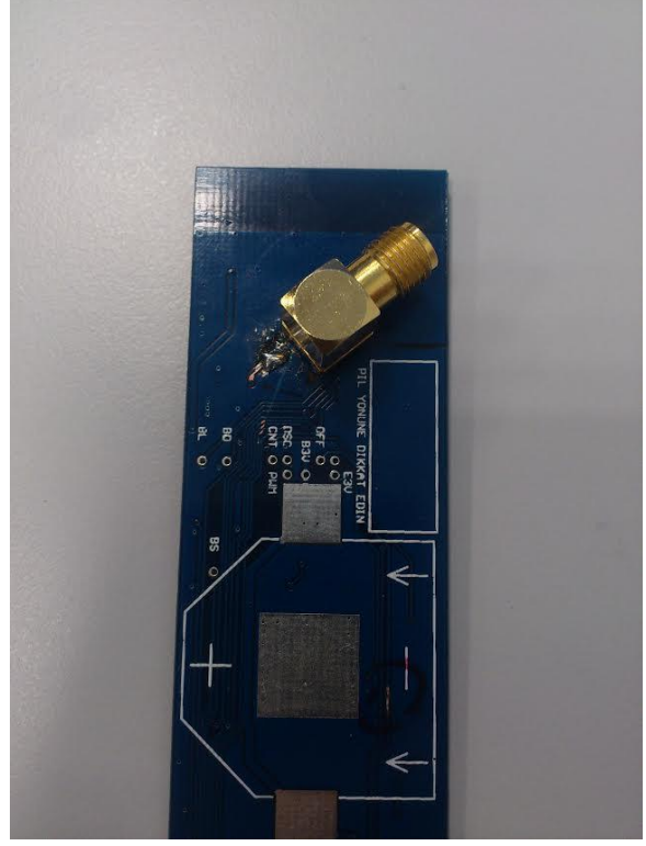
Şekil 2 - Anten ölçümü için hazırlanan PCB alt
