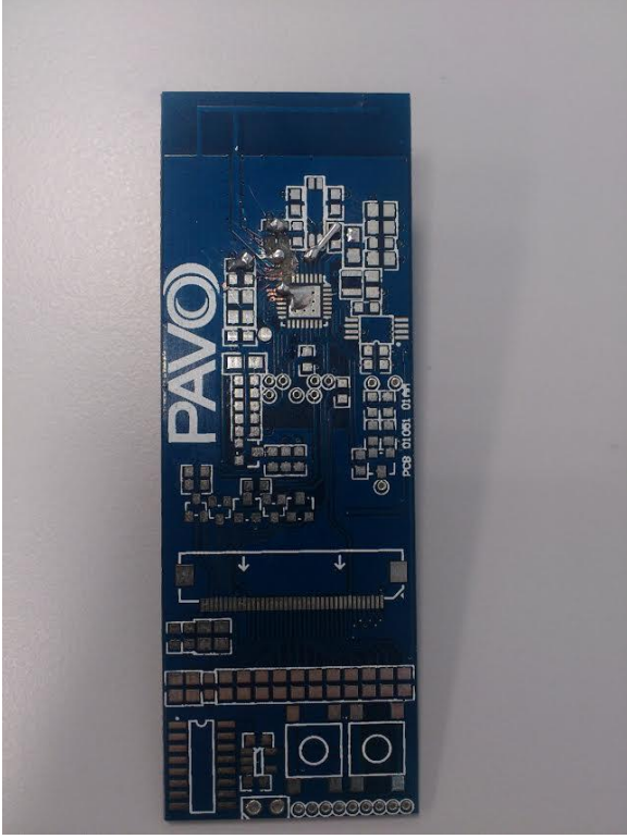
Şekil 1 - Anten ölçümü için hazırlanan PCB üst
